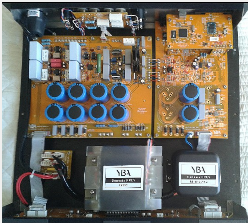
Le cœur du PRE 5 : un transformateur en double C à grains orientés Made in France. Un second transformateur est destiné à alimenter la carte de conversion numérique.
